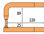
X6 Ref 050587 8 bar / 400 DaN
