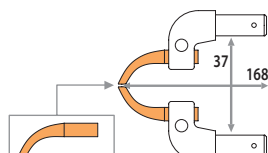
X11 Ref 051607 3 bar 150 DaN
